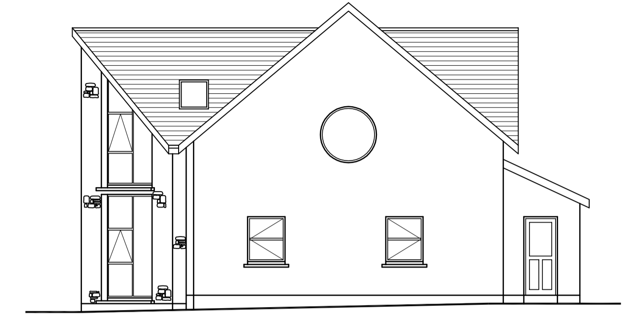
END ELEVATION
